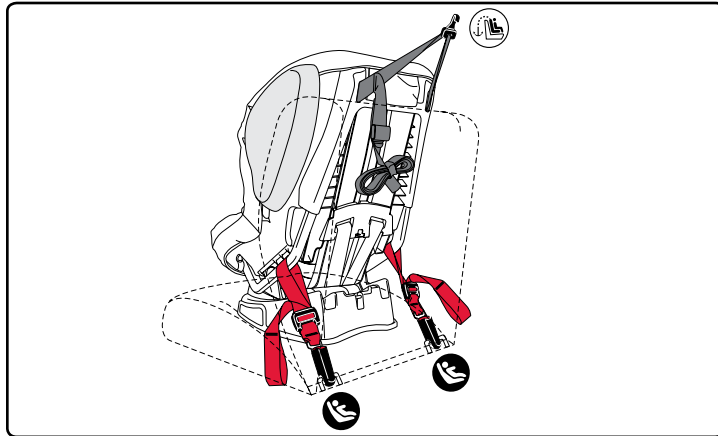
Instalación con LATCH como se indica arriba.
