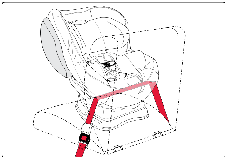
Instalación con la banda horizontal como se indica arriba.
